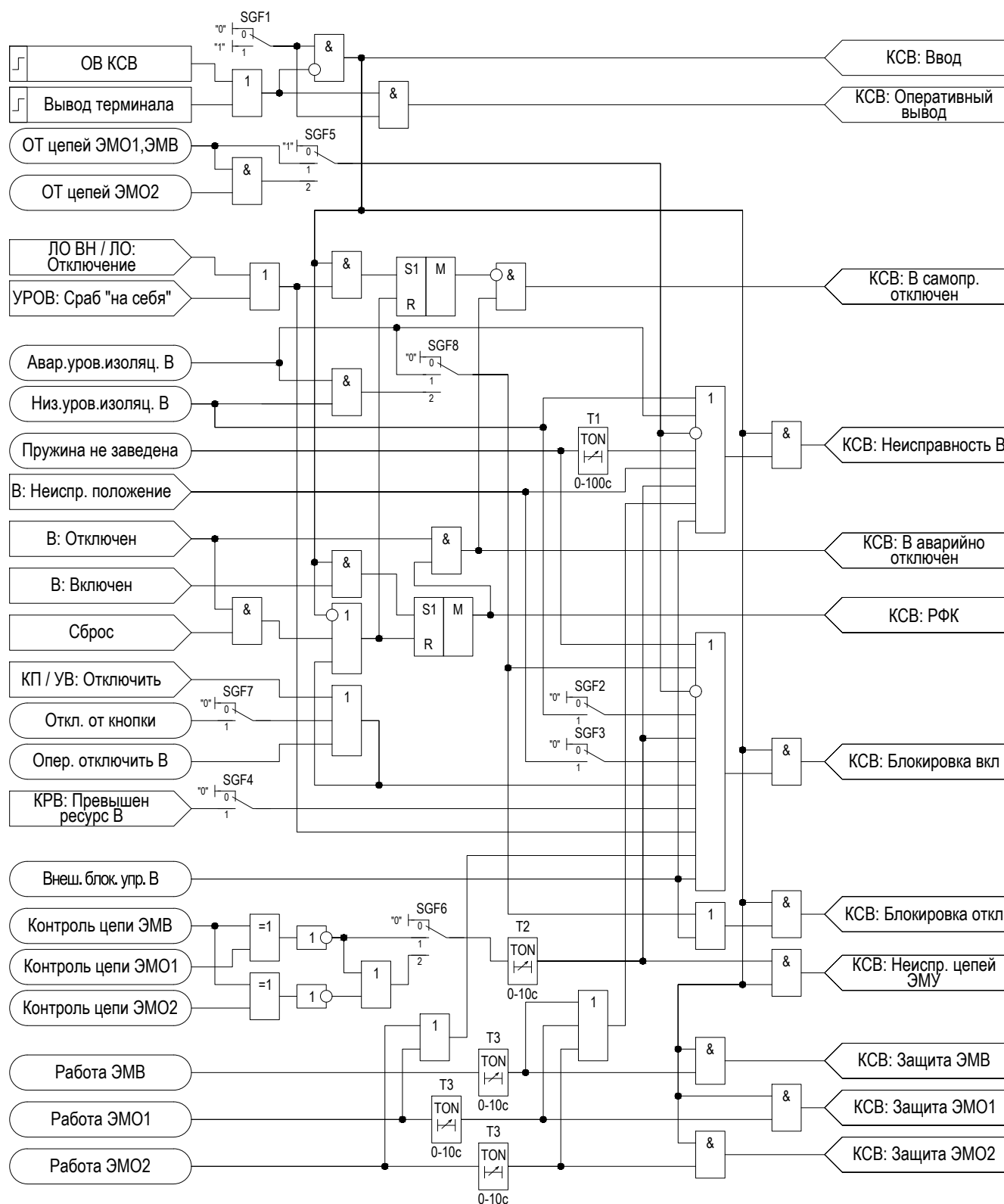
Рисунок 2.28 – Функциональная схема «КСВ»
